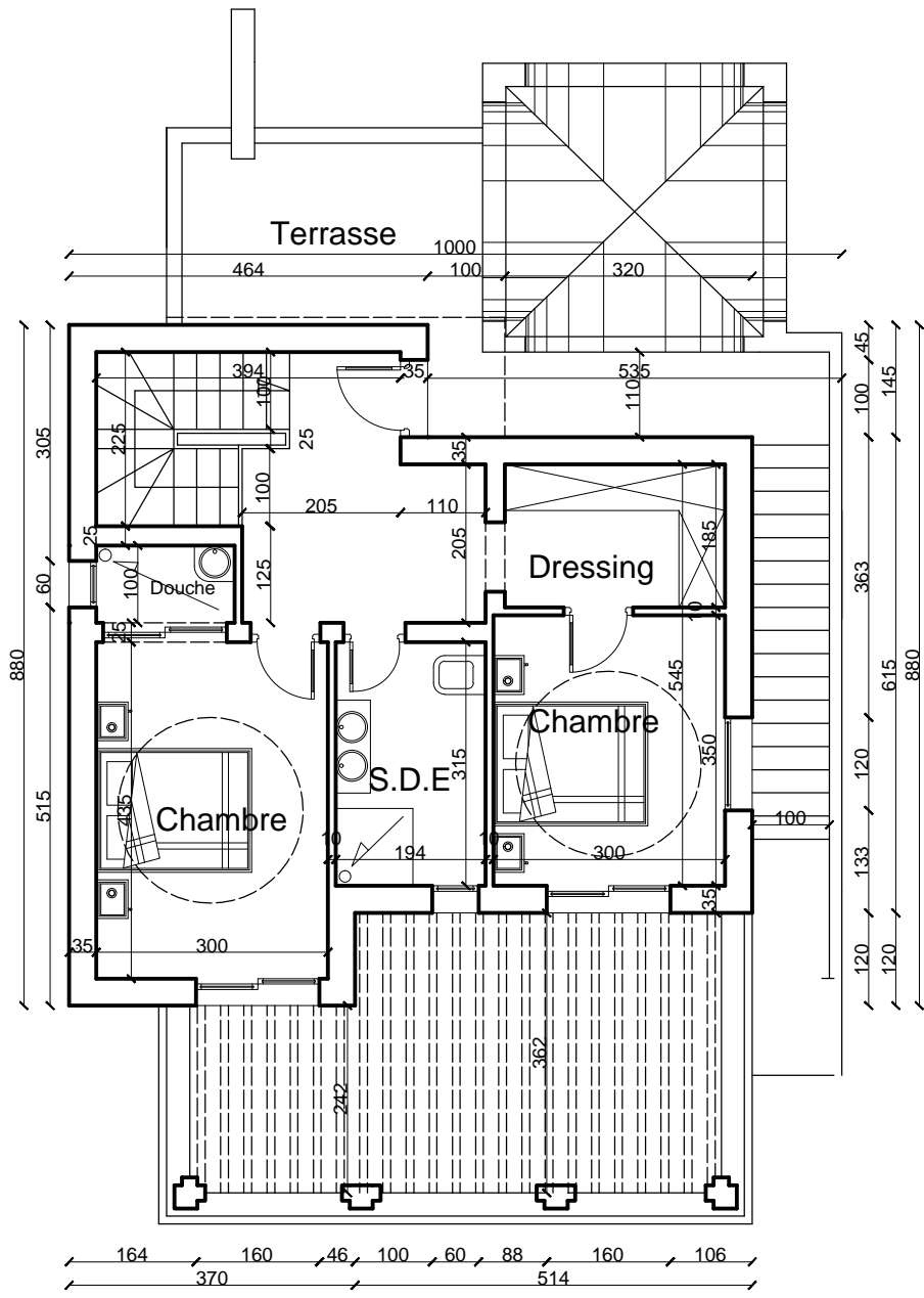
Plan Etage sc:67m 2
